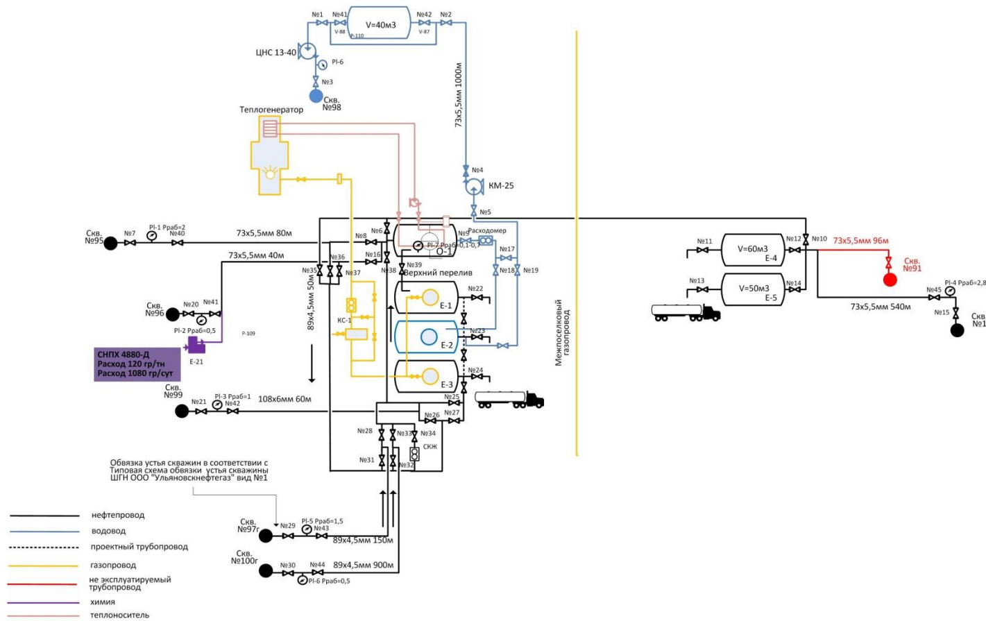
Рисунок 1 - Технологическая схема Сулакского месторождения ООО «Ульяновскнефтегаз»
