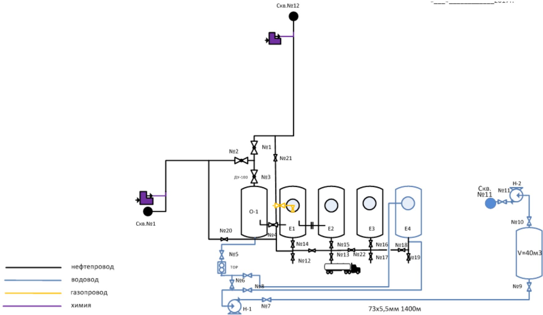
Рисунок 1 - Принципиальная схема сбора продукции скважин Славкинского месторождения
