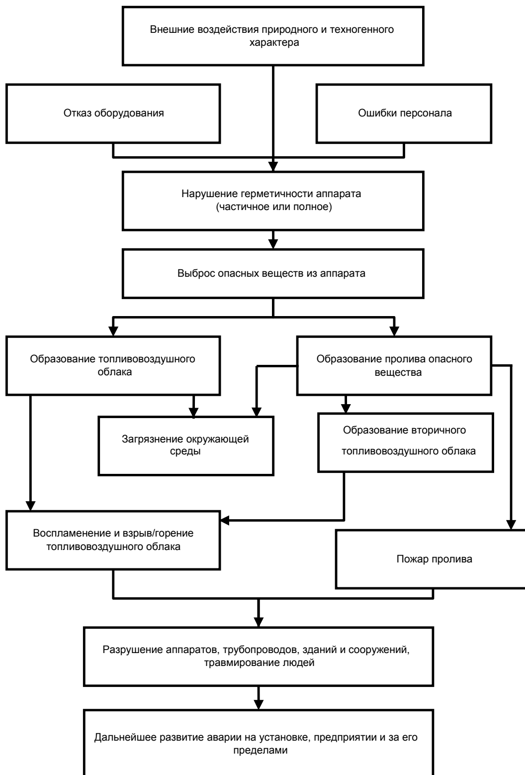
Рисунок 7 - Сценарии возможных аварийных ситуаций на объектах Славкинского месторождения ООО «Ульяновскнефтегаз»
