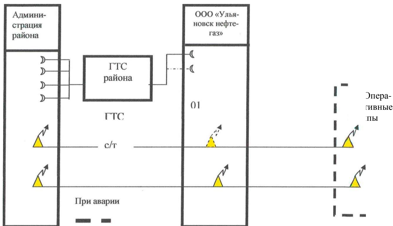
Рисунок 4 – Схема организации связи объекта (сотовой и городской телефонной)
