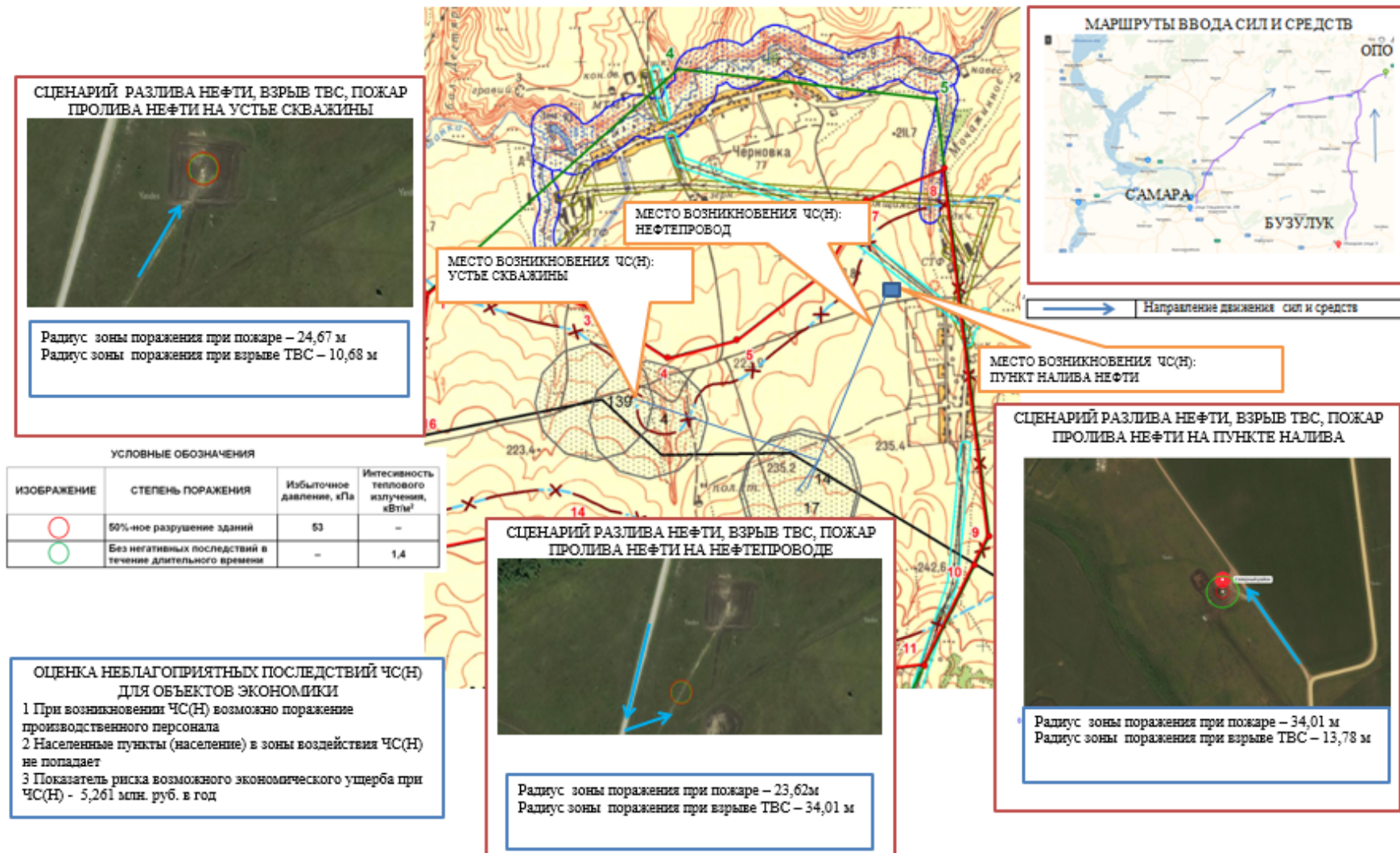
Рисунок В.2 Карта ЧС(Н) для рассматриваемых сценариев ЧС(Н) с проливом нефти на опасных производственных объектов Черновского месторождения АО «Оренбургнефтеотдача»
