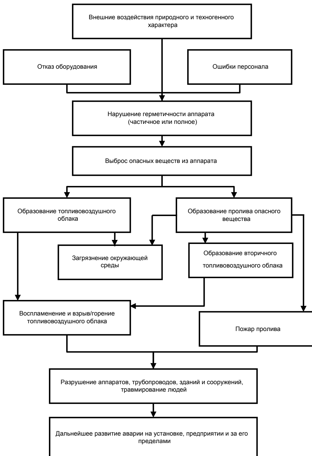
Рисунок 8 - Сценарии возможных аварийных ситуаций на объектах Ружевского месторождения ООО «Ульяновскнефтегаз»
