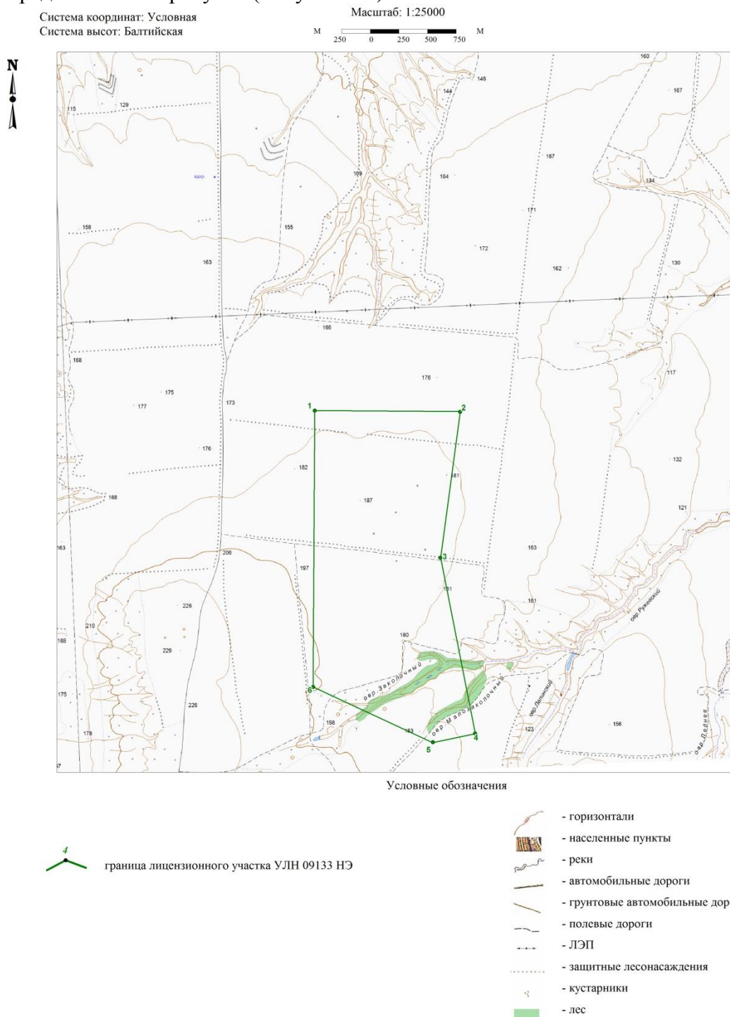
Рисунок Г.1 - Схема расположения опасных производственных объектов Ружевского месторождения ООО «УЛЬЯНОВСКНЕФТЕГАЗ»
