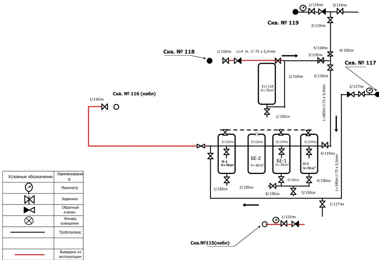
Рисунок 1 - Технологическая схема Ружевского месторождения ООО «Ульяновскнефтегаз»
