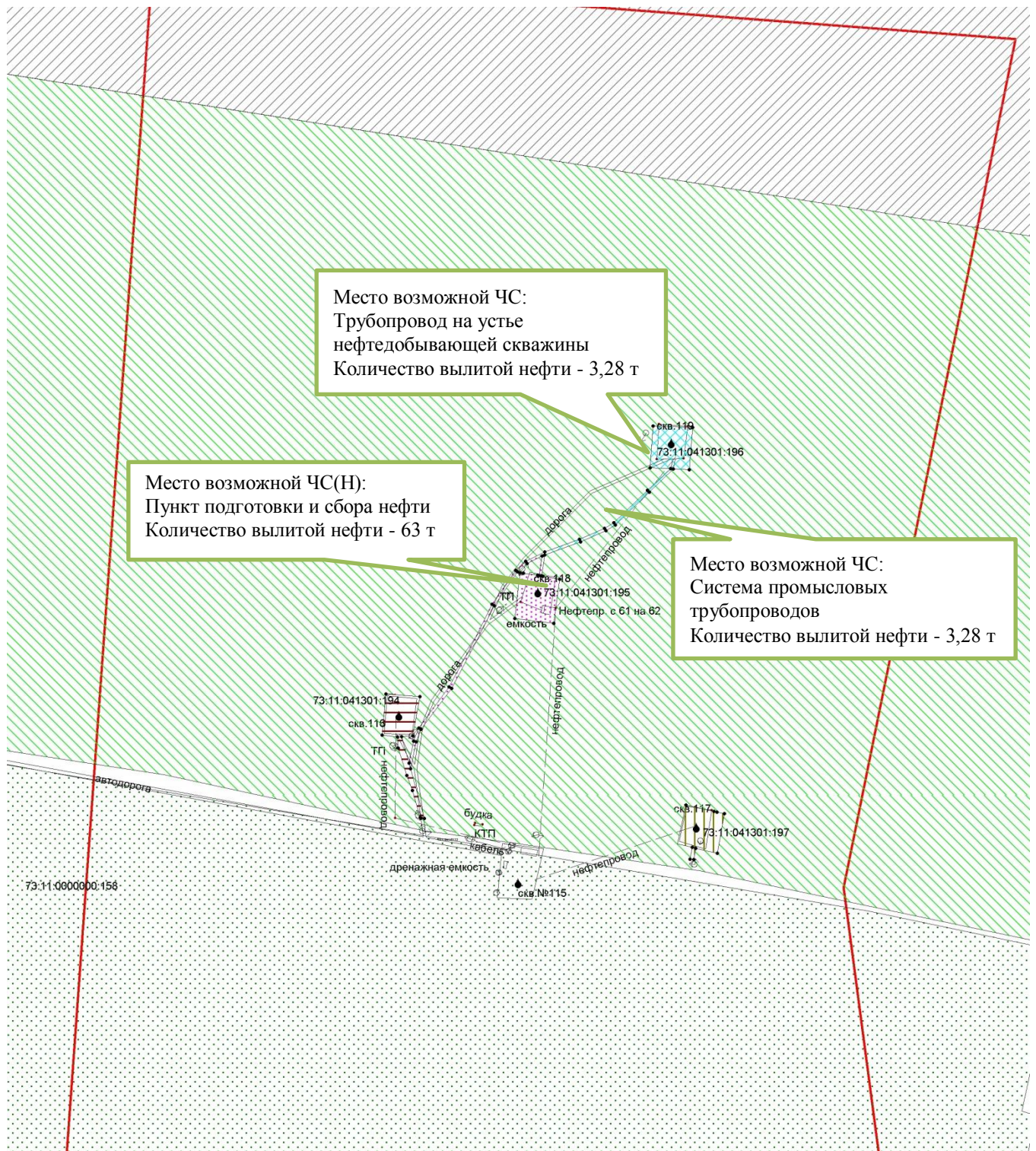
Рисунок 10 – Места возникновения ЧС на Ружевском месторождении
